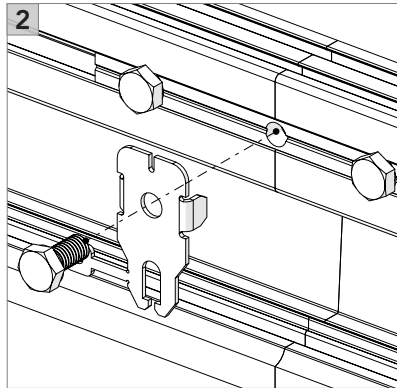
Clip d'intersection sur la jonction du profilé Hub.
