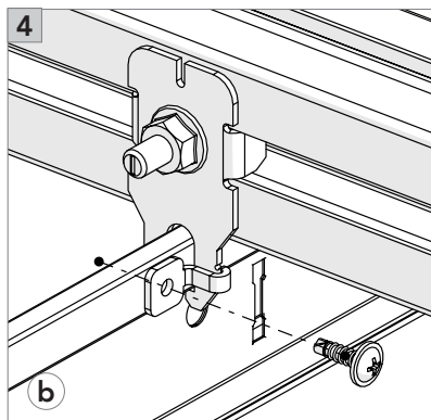
Utilisez la languette du clip d'intersection et fixez-la aux profilés porteurs T24 (2 par profilé porteur - à chaque extrémité) à l'aide d'une vis autoforeuse.
